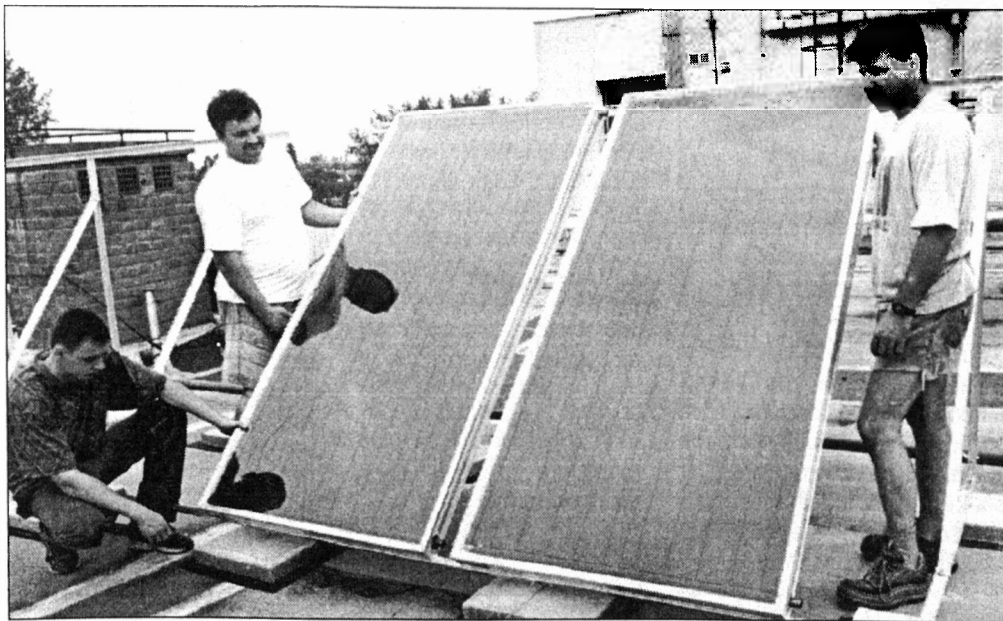
Napkollektorokat helyeztek el a Munkácsy Mihály Szakközépiskola leány kollégiumának tetején. Felvételünk készítésekor az egyik acél keretszerkezetre éppen iker-napcellát rögzítettek fel. A beruházást – melyet a gyulai képviselő-testület is támogatott – az intézmény fenntartója, a Békés Megyei Önkormányzat finanszírozza pályázaton nyert pénzből. A fejlesztéssel nemcsak energiát takaríthat meg az iskola, a beruházás környezetvédelmi célokat is szolgál
